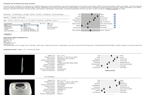
Fig. 4 : Interface Web
